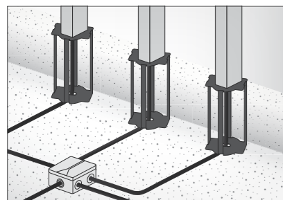
Abzweigkasten/Erdstück: distribution box/anchorage unit:
