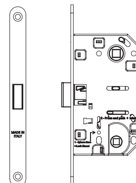
Foro nottolino Privacy set hole
