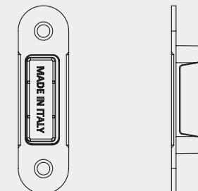
Incontro con piastrina per serratura magnetica Striking plate with platelet for magnetic lock Cod. 181003
